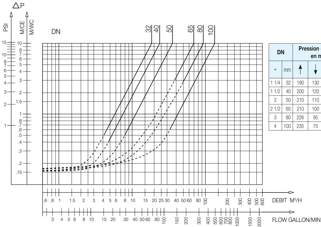
802L - Abaque de pertes de charge
